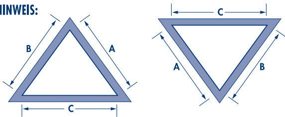
GESCHLOSSEN MIT ÖSE
